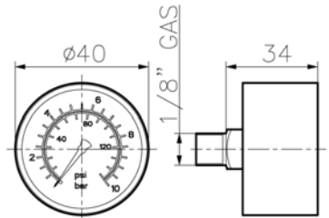
Return filter indicator Scale: 0÷10 bar - VR Type
